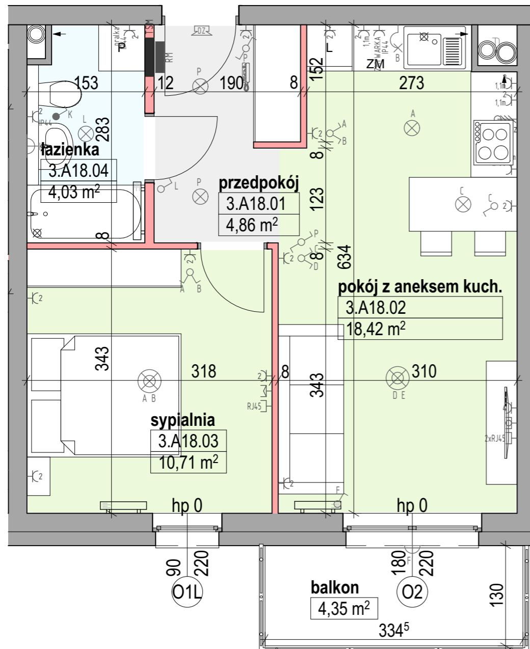
RZUT MIESZKANIA
