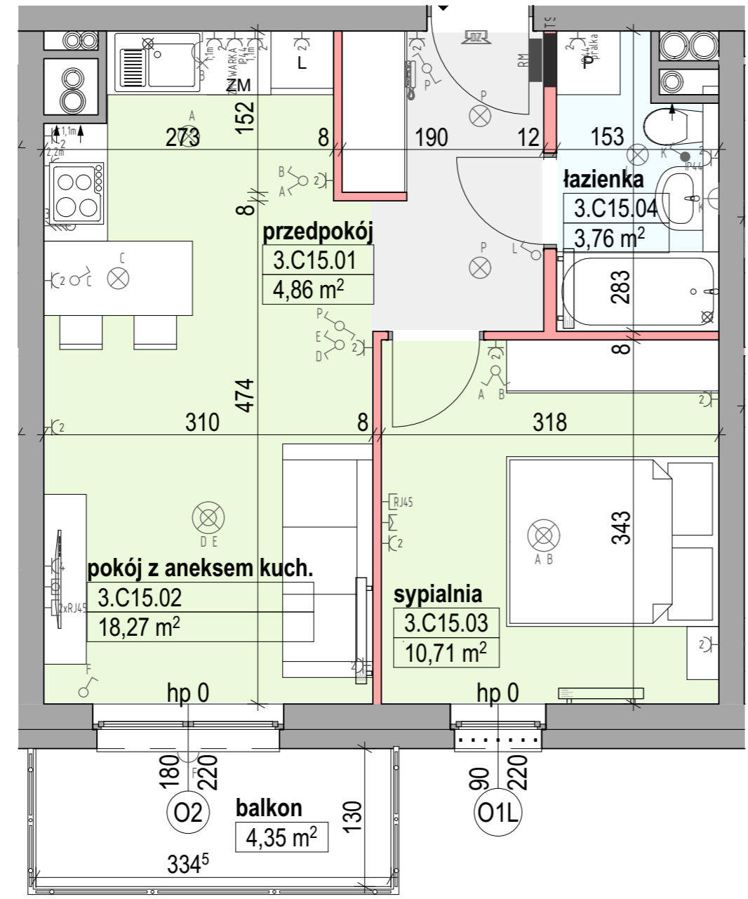
RZUT MIESZKANIA
